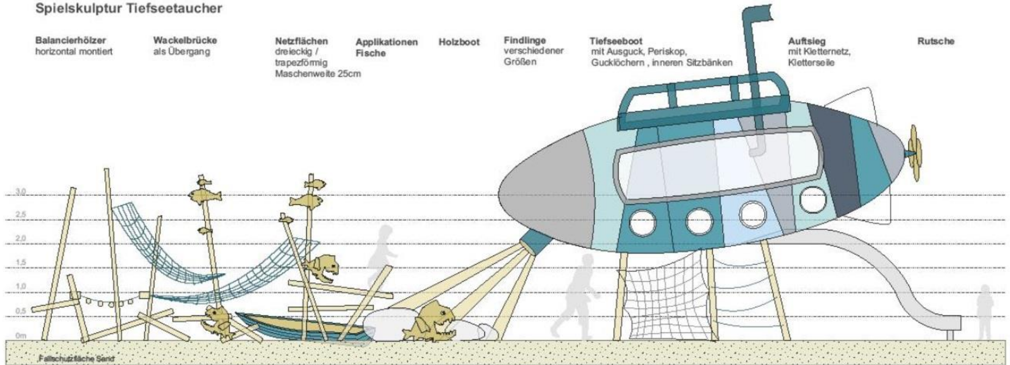
Schnittansicht Spielfunktionen
